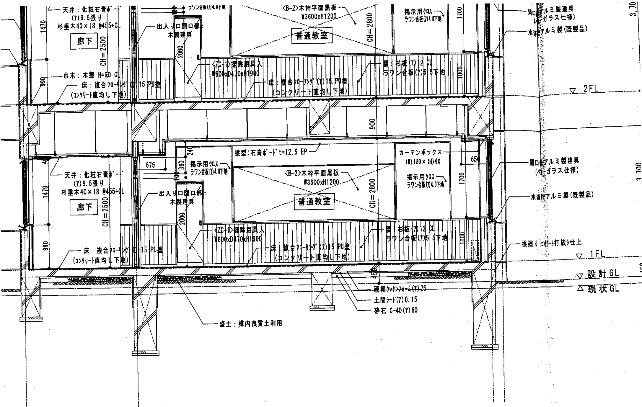
普通教室廻り矩計詳細図 S=1/50
