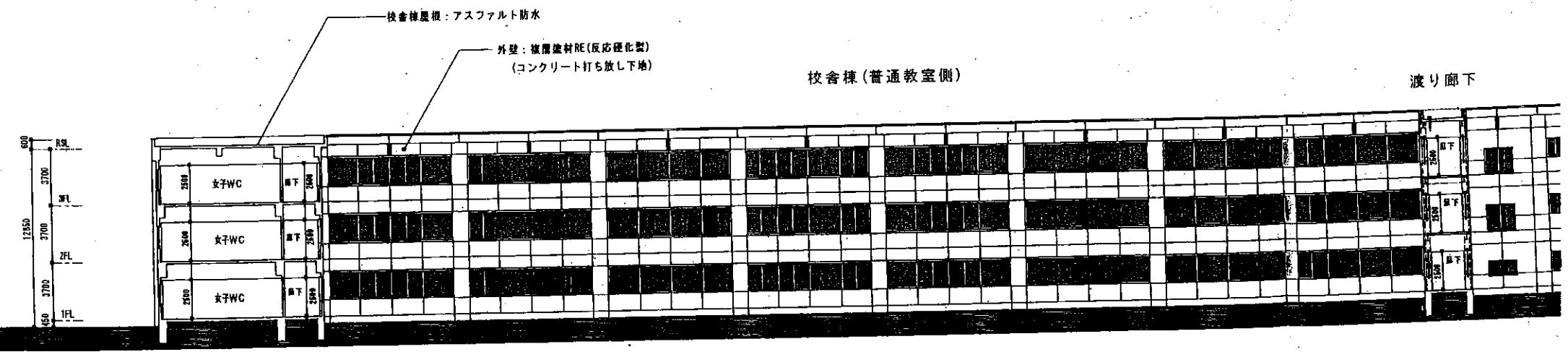
中庭南側立面図 1/250
